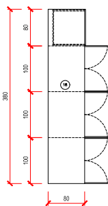
18 – BANCADA + ARMÁRIO DE BANCADA 3 módulos com 2 portas 1 prateleira + 1 módulo 4 gavetas 380x80x90 (CxLxA)
