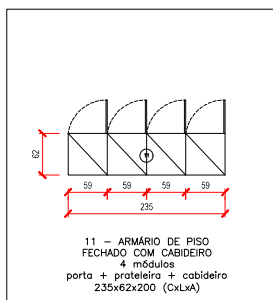
DETALHAMENTO MOBILIÁRIO ANTE SALA 1
