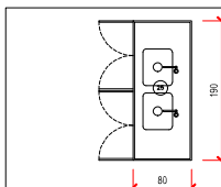
25 – BANCADA COM 2 CUBAS + ARMÁRIO DE BANCADA 4 portas acesso ponto hidráulico 190x80x90 (CxLxA)
