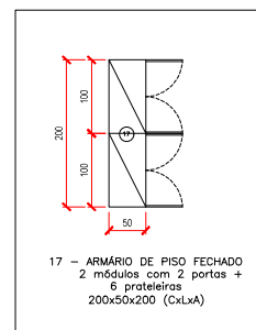
DETALHAMENTO MOBILIÁRIO SALA GASES NOBRES
