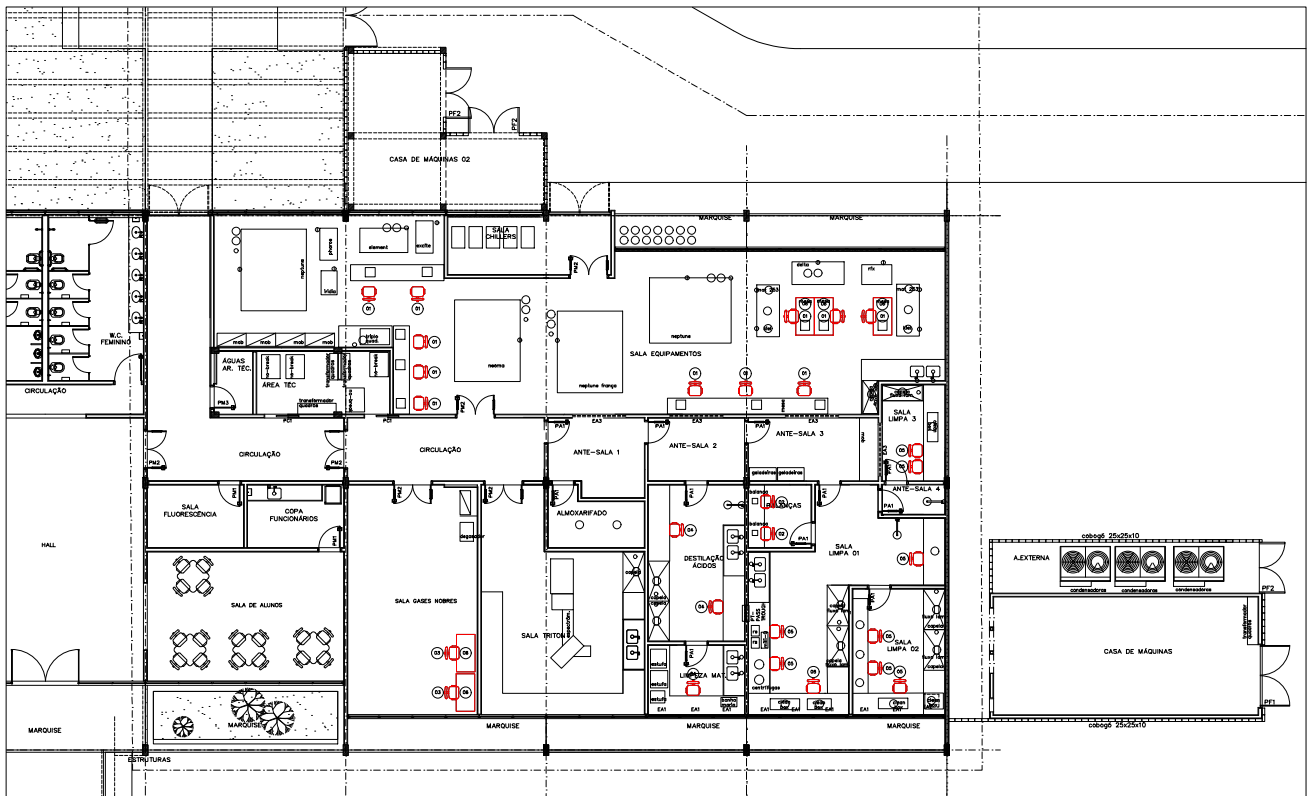
PLANTA DE LOCAÇÃO DE MOBILIÁRIO
