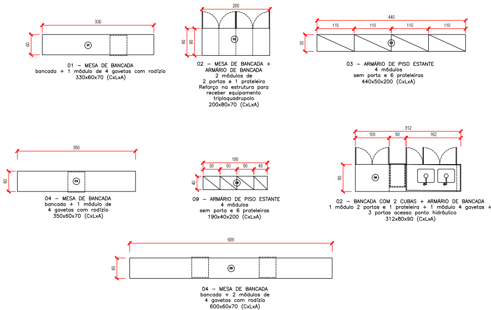
DETALHAMENTO MOBILIÁRIO SALA EQUIPAMENTOS
