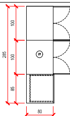
21 – BANCADA COM CUBA + ARMÁRIO DE BANCADA 2 módulo 2 portas e 1 prateleira + 1 módulo 4 gavetas 285x80x90 (CxLxA)
