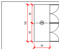
23 – BANCADA + ARMÁRIO DE BANCADA 2 módulos com 2 portas 1 prateleira 190x80x90 (CxLxA)
