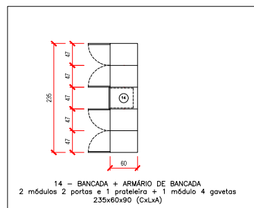
DETALHAMENTO MOBILIÁRIO ANTE SALA 3
