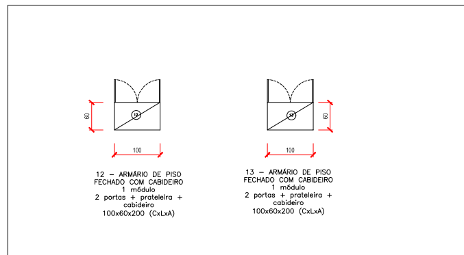
DETALHAMENTO MOBILIÁRIO ANTE SALA 2
