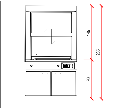
VISTA CAPELA REFERENCIA
