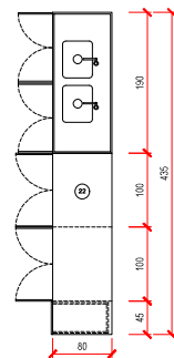
22 – BANCADA COM 2 CUBAS + ARMÁRIO DE BANCADA 2 módulo 2 portas e 1 prateleira + 4 portas acesso ponto hidráulico 435x80x90 (CxLxA)
