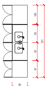
20 – BANCADA COM 2 CUBAS + ARMÁRIO DE BANCADA 2 módulo 2 portas e 1 prateleira + 4 portas acesso ponto hidráulico 377x80x90 (CxLxA)
