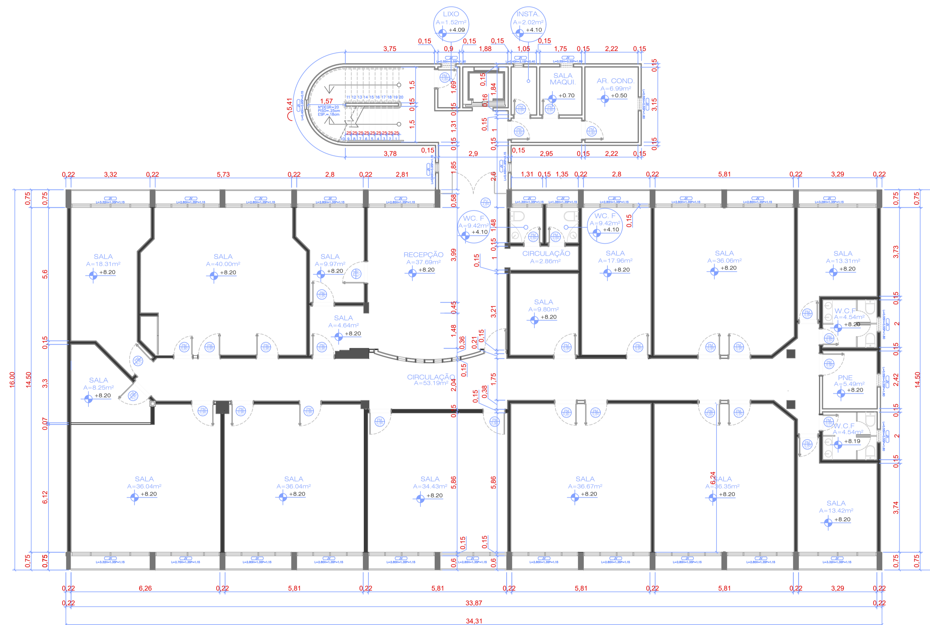
PLANTA BAIXA 2º PAVIMENTO ESCALA 1:100
