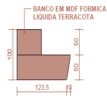
CORTE BANCO - 01 ESC. 1 : 50
