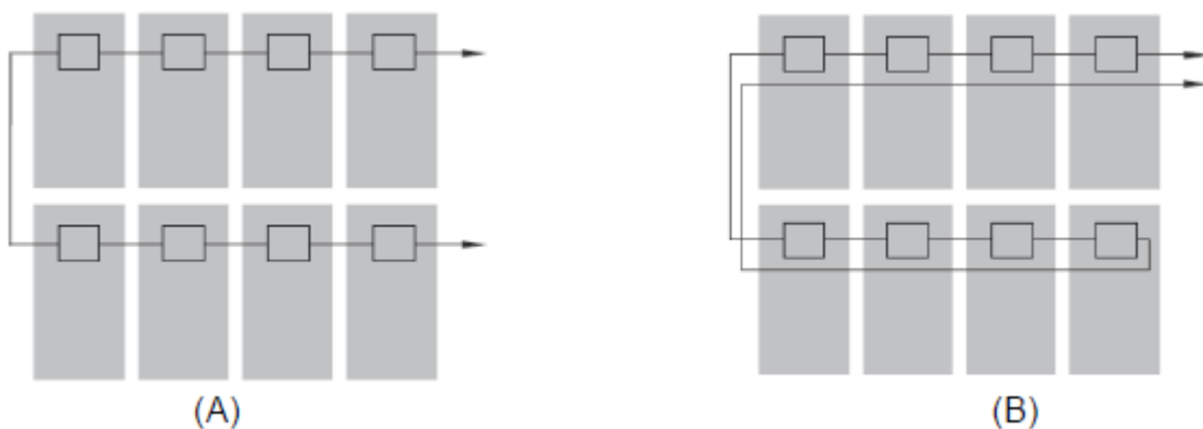
Figura 2: Método de instalação dos cabos CC. (a) Método não permitido para a instalação fotovoltaica (b) Método a ser considerado na instalação fotovoltaica, para minimizar indução de descargas atmosféricas
